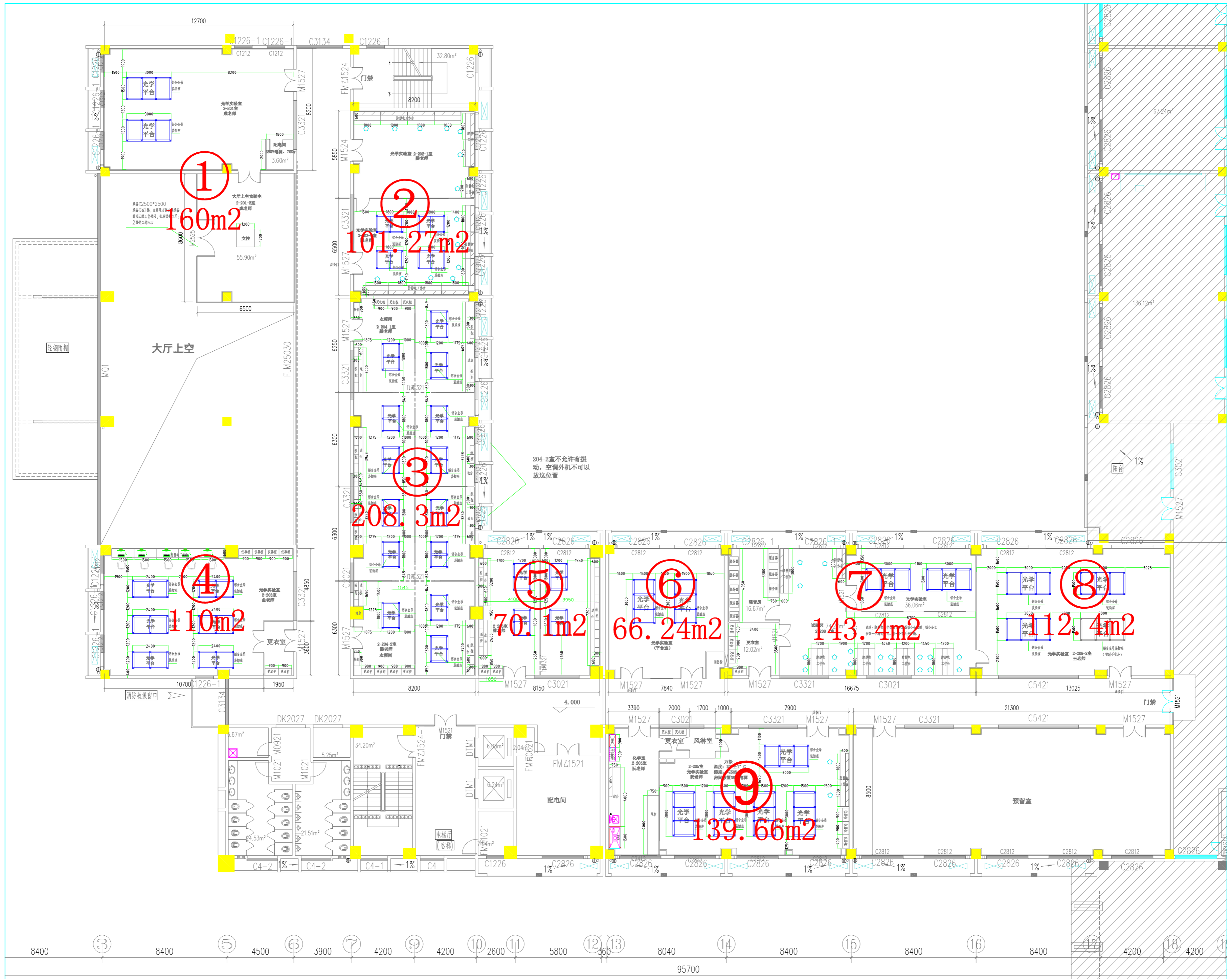
二层平面布置图 1:100
